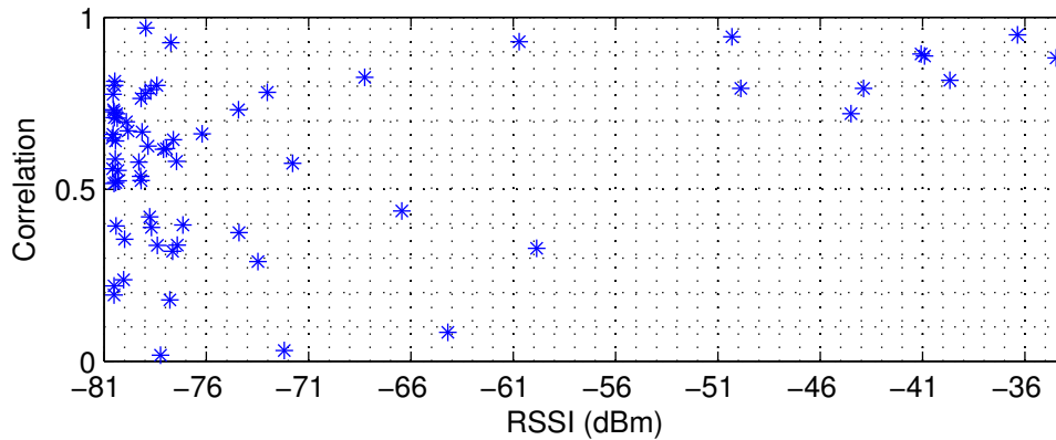
Fig. 3. Correlation vs RSSI.
